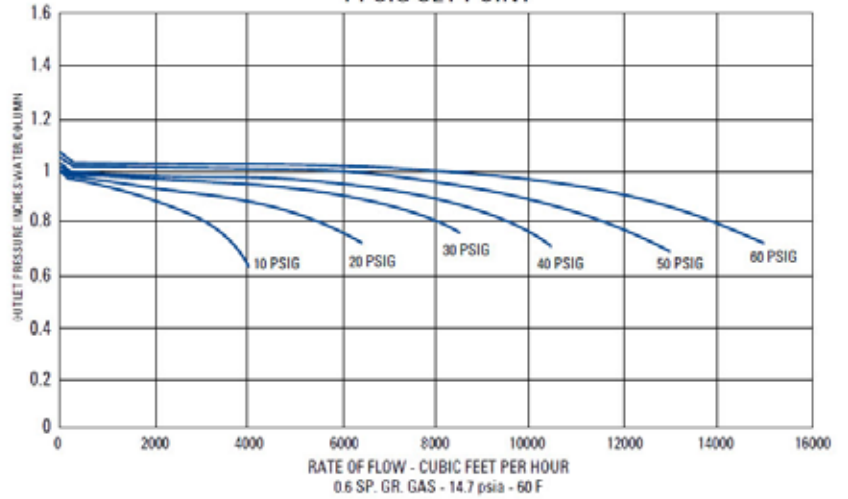
B38 IM REGULATOR PERFORMANCE 1 PSIG SET POINT
