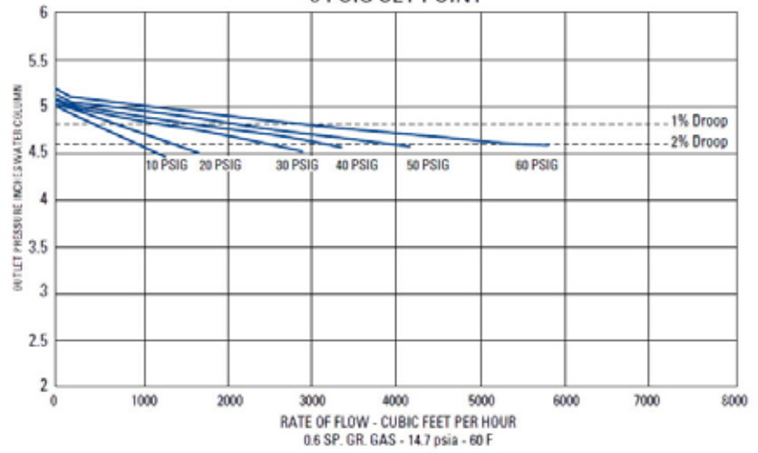
B38 IM REGULATOR PERFORMANCE 5 PSIG SET POINT
