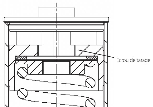
Ecroûs de tarage ressort de régulation : No. 20231000
