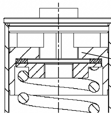
Регулировочный ключ для юстировочного винта: № 20231000
