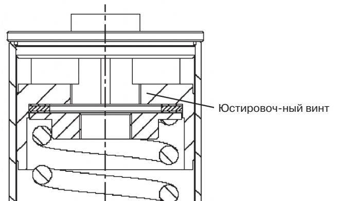
Регулировочный ключ для юстировочного винта: № 20231000
