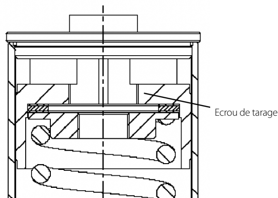
Ecrous de tarage ressort de régulation : No. 20231000
