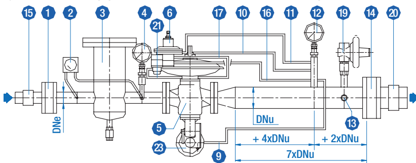
Installationsbeispiel mit Regelgerät und integriertem SAV
