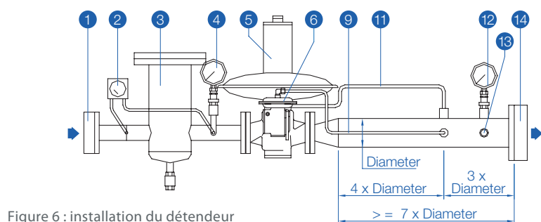
Figure 6 : installation du détendeur
