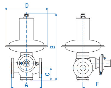
RB 4000 und SAV 8500
