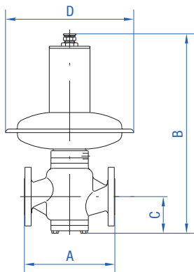
Regelgerät RB 4000 - DN 25, 40, 50 & 80
