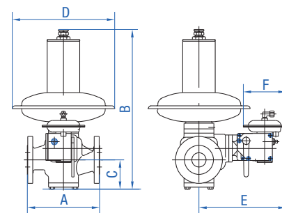
RB 4000 und SAV 8600 DN 25, 40, 50 & 80
