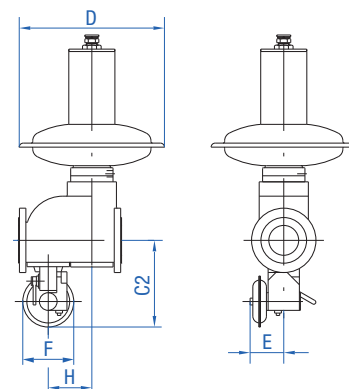
RB 4000 und SAV 8600 DN 100
