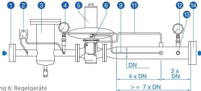
Zeichnung 6: Regelgeräte Installationsbeispiel
