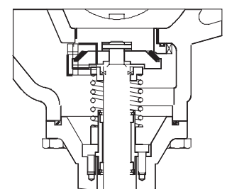
Fig. 9 SAV Baugruppe
