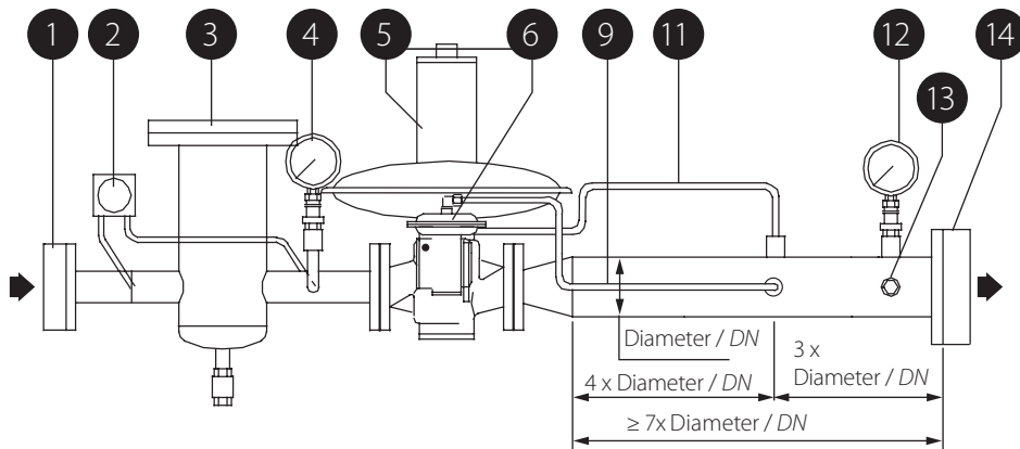
Fig 6 - Regulator installation / Zeichnung 6: Reglergeräte Installationsbeispiel
