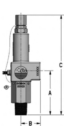
M (Micro) Body
