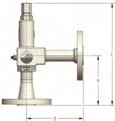
M (Micro) Body
